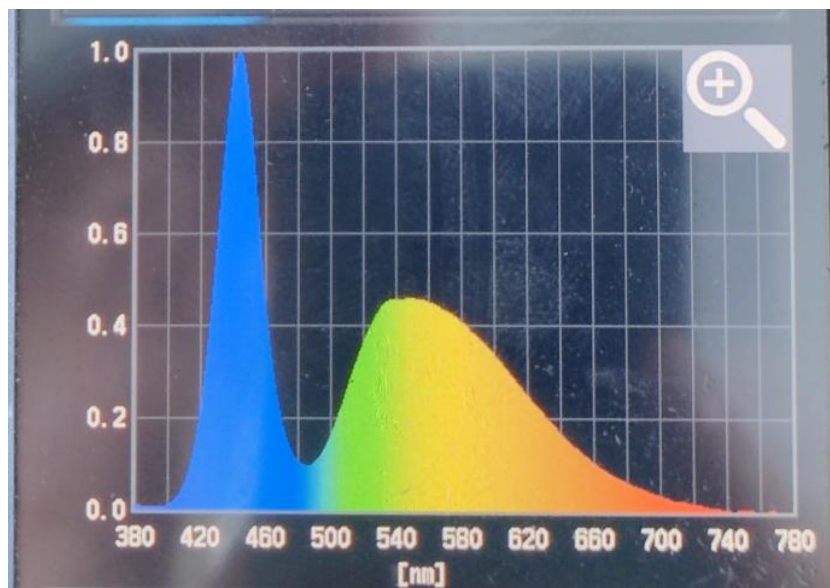
图解：在建议 5A 电流下的典型光谱(8100K)
